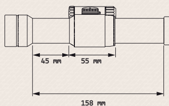
Aimpoint® 9000L
